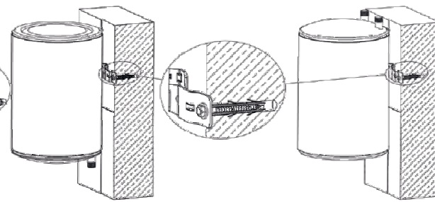
Кріплення моделей з установкою під мийку: PC 10SB, PC 15S, PC 15SB
