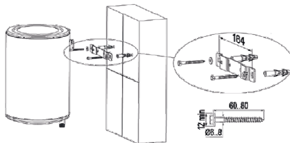
Кріплення моделей РС
