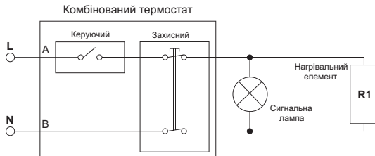
Рисунок 6. Схема електрична для моделей: N4, N4L, N4s, D400-1-M, PC, D443-1-M
