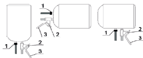
А - Вертикально Б - Горизонтально В - Горизонтально
