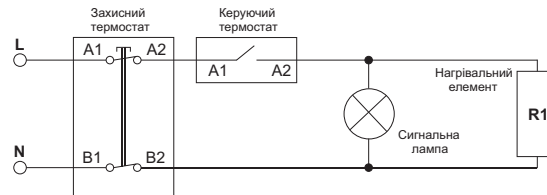
Рисунок 7. Схема електрична для моделей: D400-2-B, D325-2-BC, D400-1-BC, D400-2-BC, D443-2-BC
